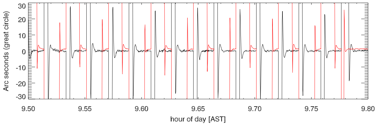
Az, Za tracking error blowup
