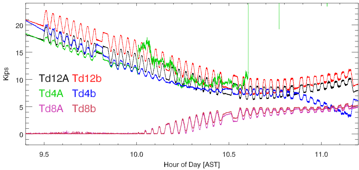
tiedown Tensions
