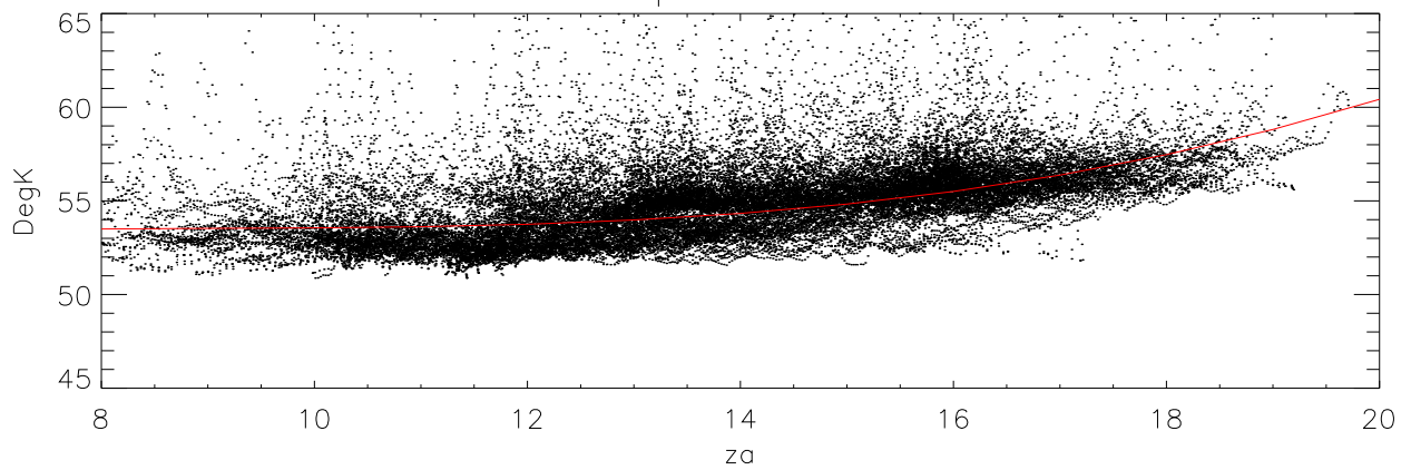
PolA data Epoch 2 data and fit.
