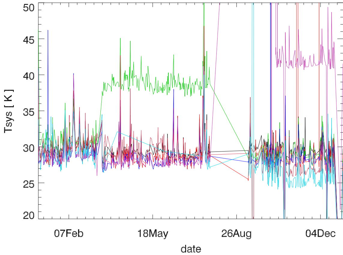
Alfa Tsys yr:2011 PoIA
