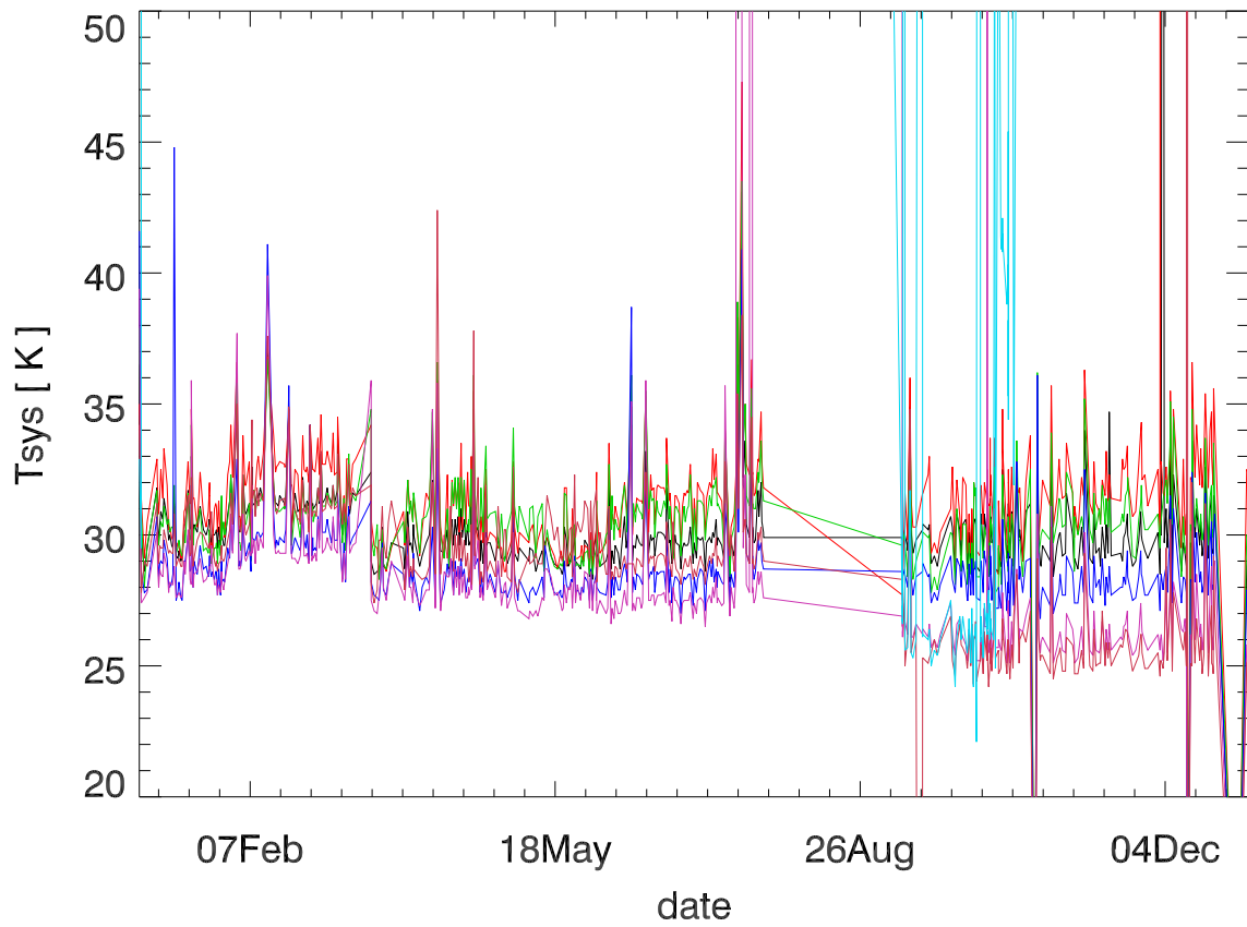
Alfa Tsys yr:2011 PoIB
