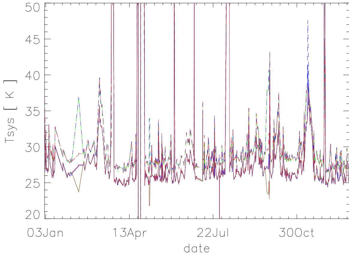
CBAND Tsys yr:2010
