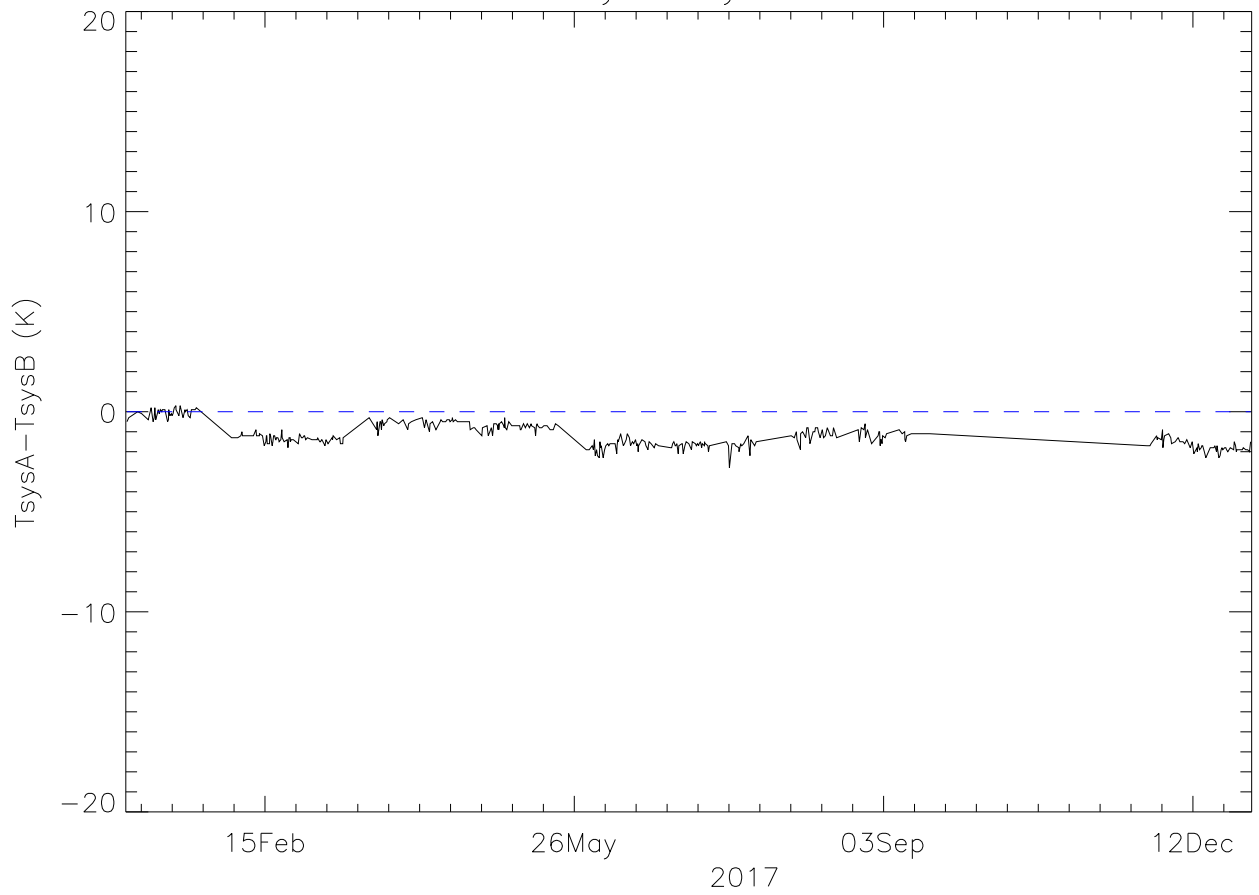
sbh T_{\text{sysA}} - T_{\text{sysB}} 2017
