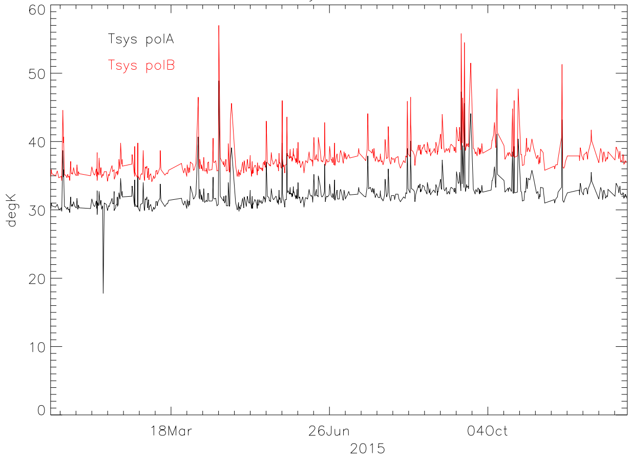
xb TsysA-TsysB 2015
