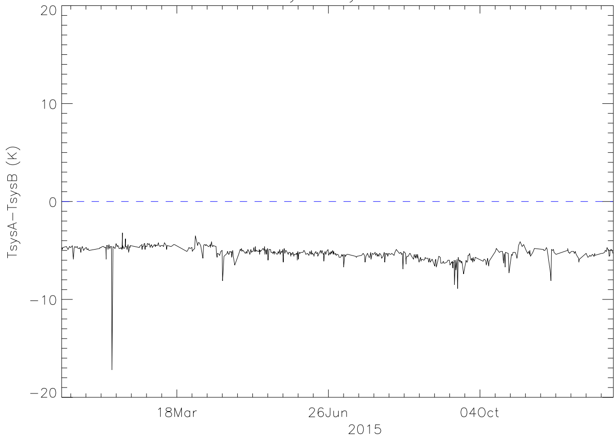
xb TsysA-TsysB 2015
