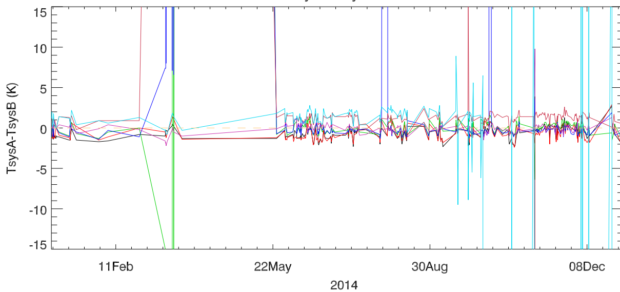
alfa TsysA-TsysB 2014
