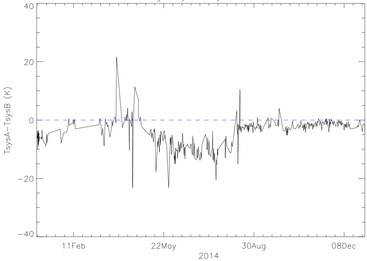
430gr TsysA - TsysB 2014
