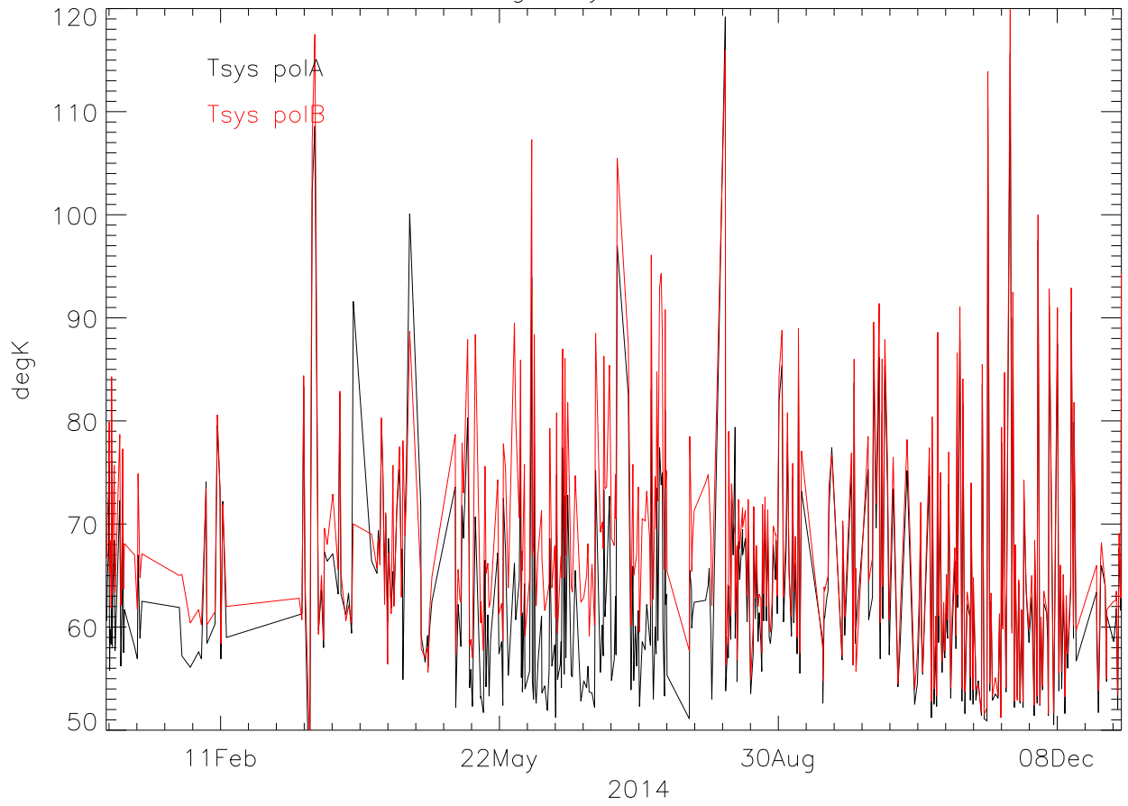
430gr TsysA - TsysB 2014
