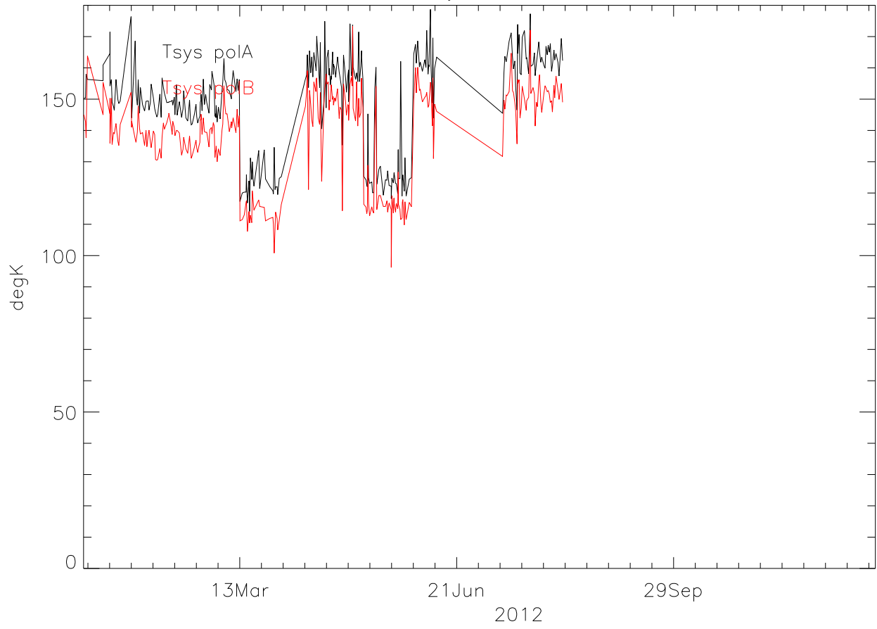
800 TsysA-TsysB 2012
