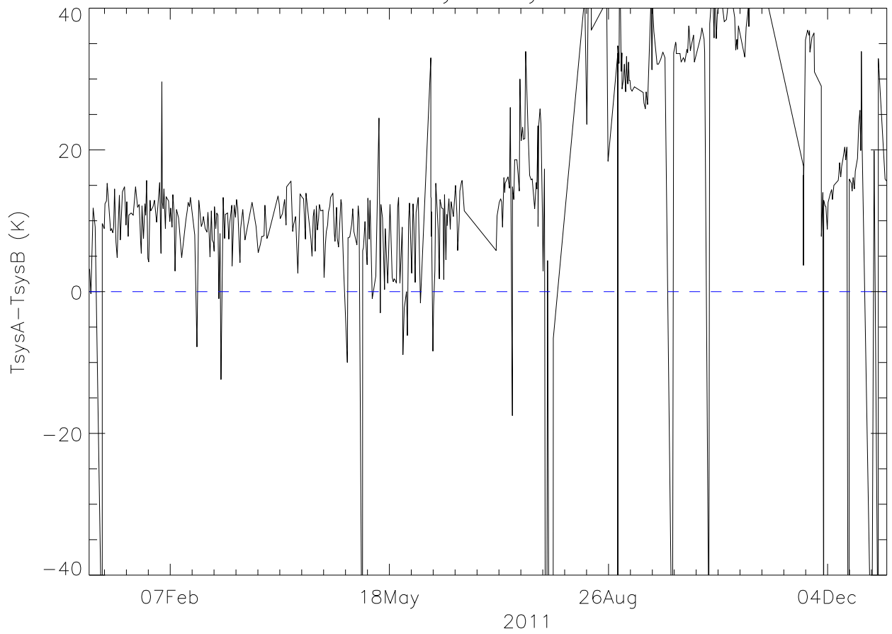
430ch TsysA-TsysB 2011
