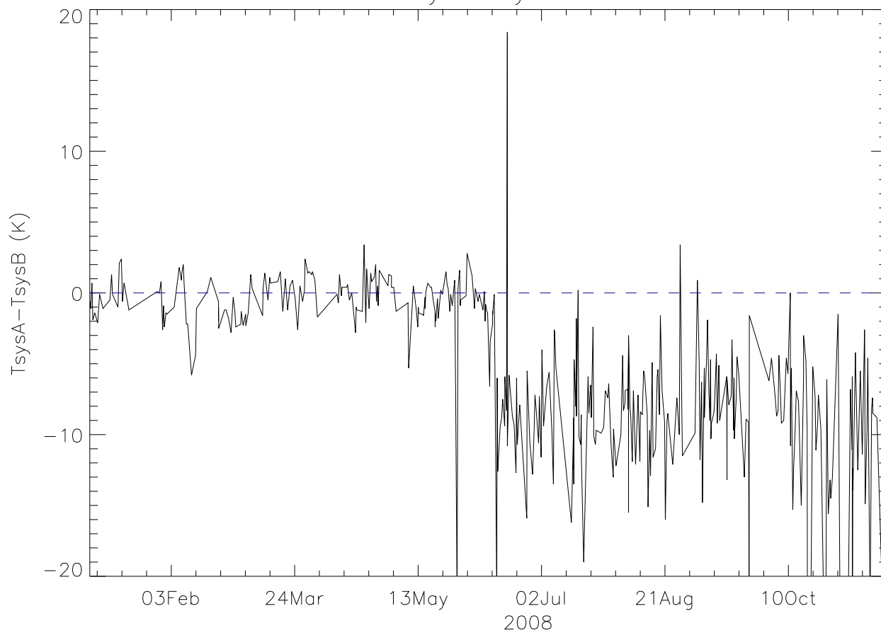
327 TsysA - TsysB 2008
