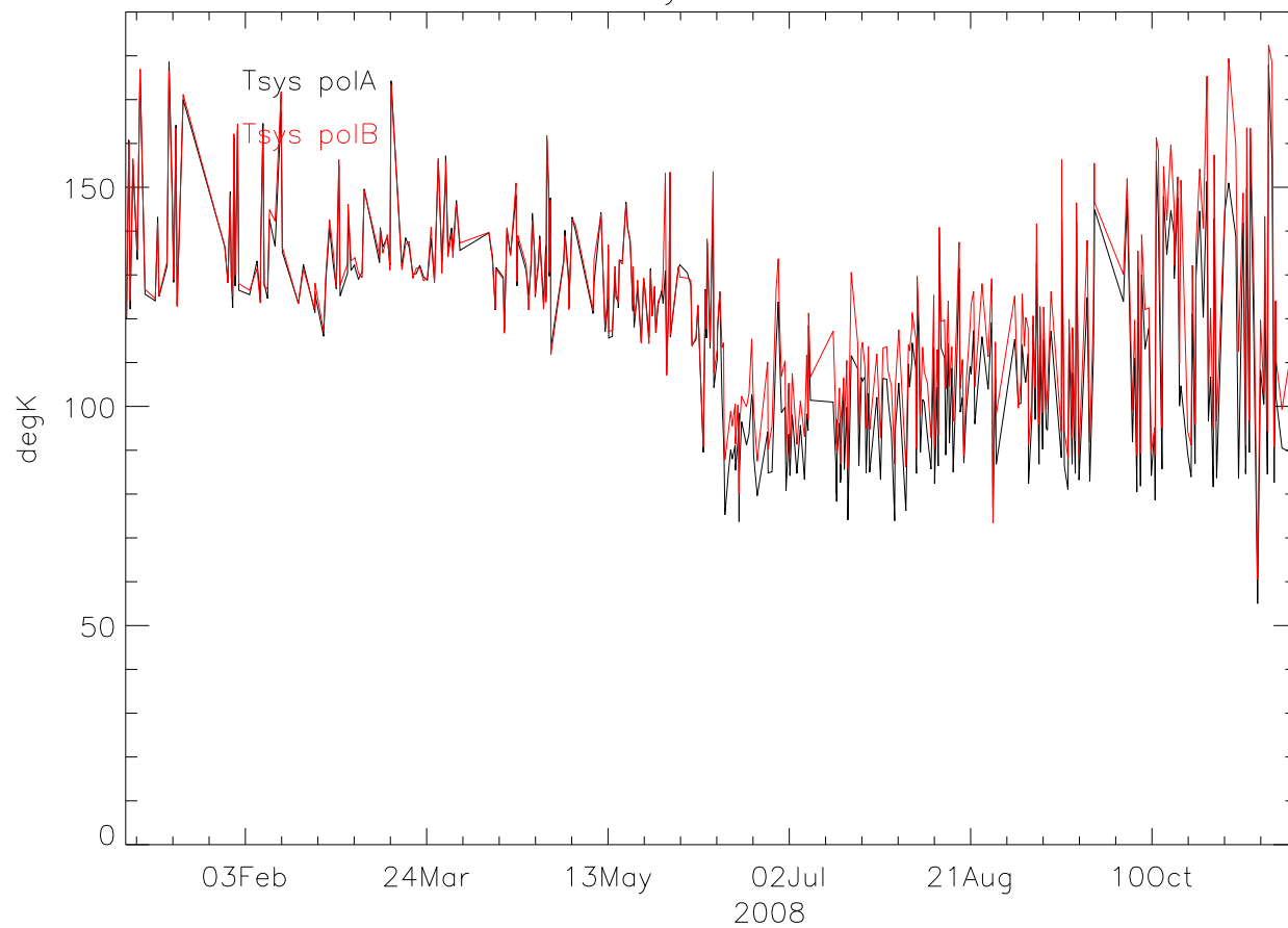
327 TsysA - TsysB 2008
