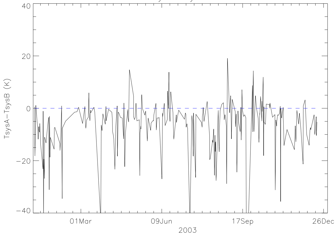
610 TsysA-TsysB 2003
