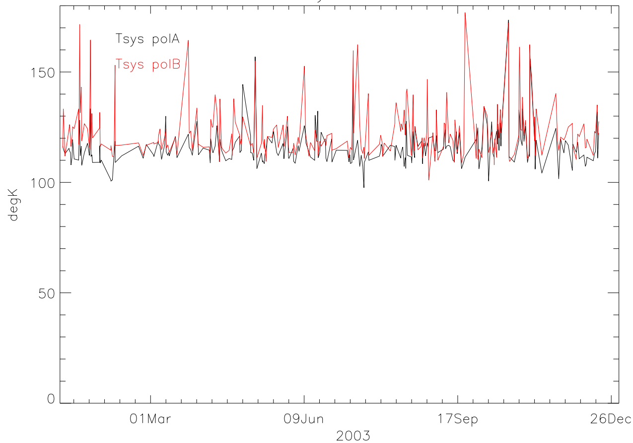
610 TsysA-TsysB 2003
