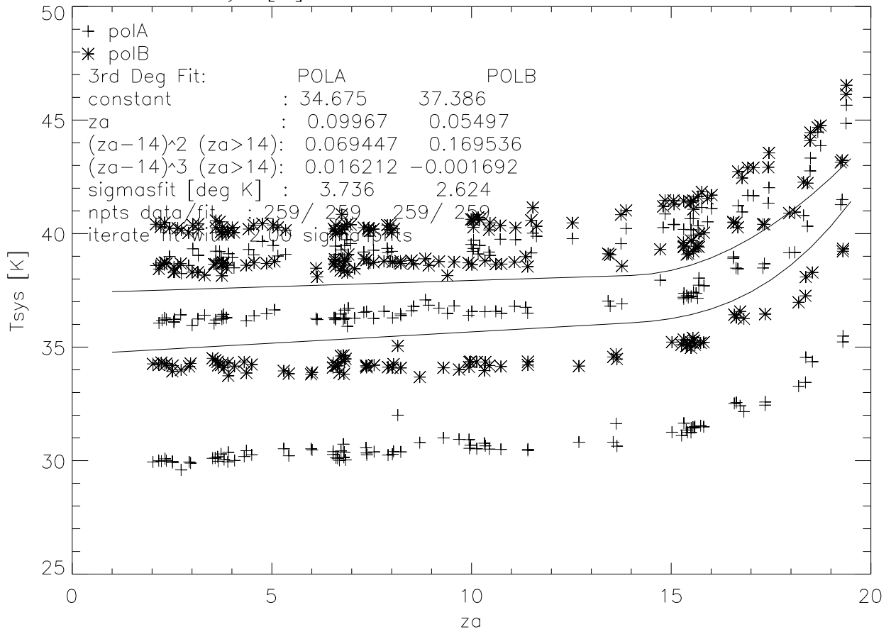
Tsys [K] vs Za CB 4-6 Ghz , APR-JUL00
