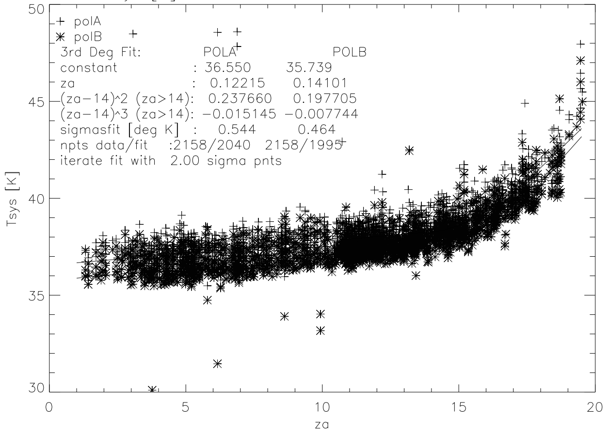
Tsys [K] vs Za LBW 1300-1425 MHZ, APR-JUL00
