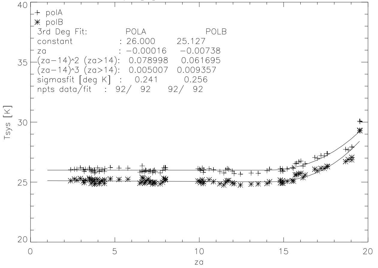
Tsys [K] vs Za SBN, APR-JUL00
