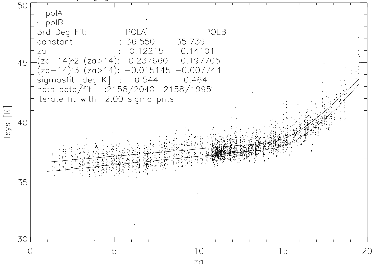
Tsys [K] vs Za LBW 1300-1425 MHZ, APR-JUL00
