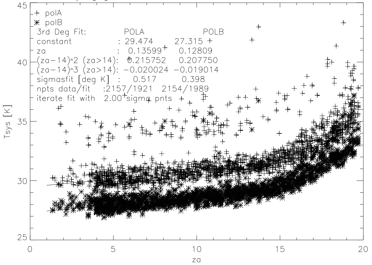
Tsys [K] vs Za LBN 1400-1425 MHz, APR-JUL00
