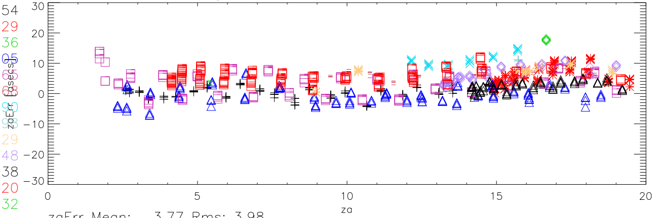
jun12-dec12. cb rcvr. za error vs za
