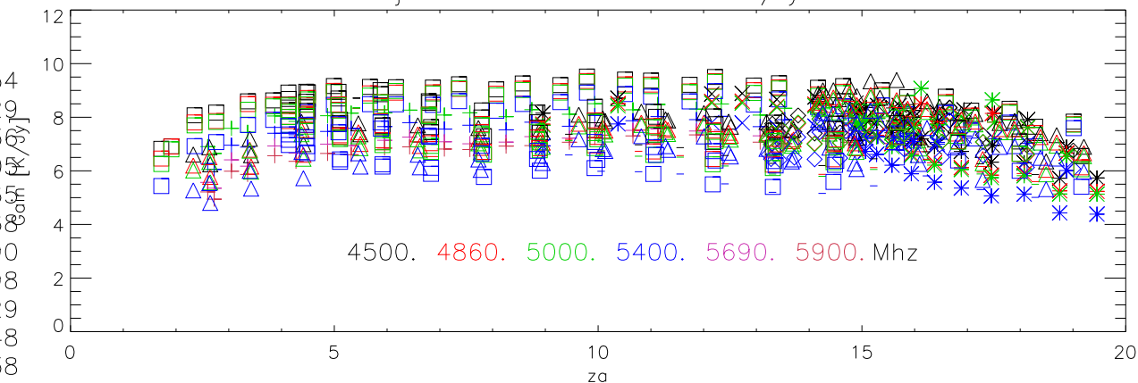
jun12-dec12. cb rcvr. Gain K/Jy
