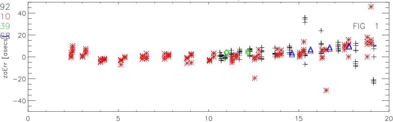
01mar19 to 31mar19 lbw 252 pnts. za error vs za
