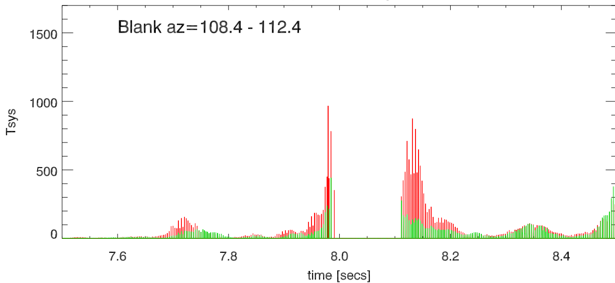
PuntaBorinquen blanking toward AO
