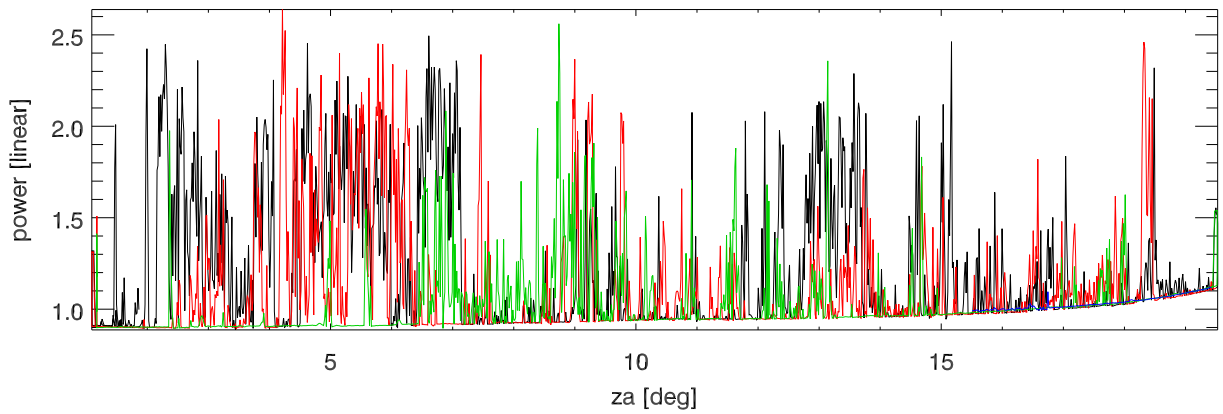
bm0 polA tp vs za.1300 Mhz band
