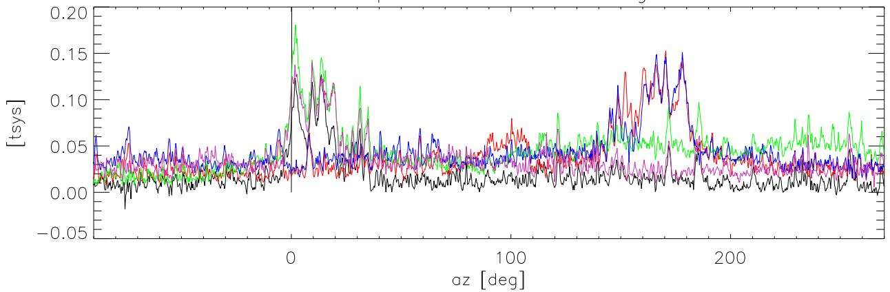
28oct10 321.90 az dependence for 5 az swings. fmstation:107.3
