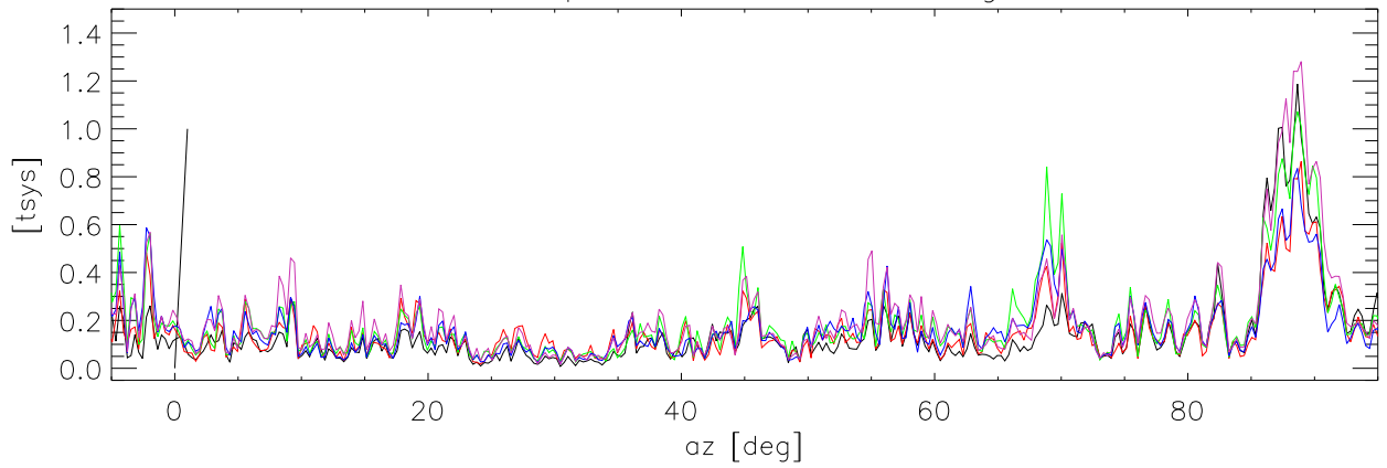
28oct10 312.30 az dependence for 5 az swings. fmstation:104.1
