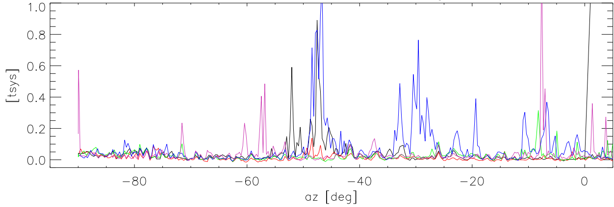
28oct10 321.90 az dependence for 5 az swings. fmstation:107.3
