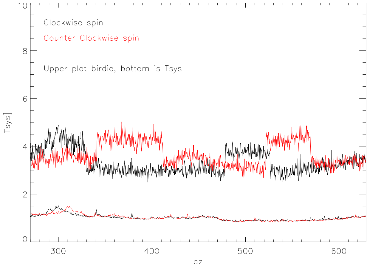
11oct05 310.35 birdie vs az
