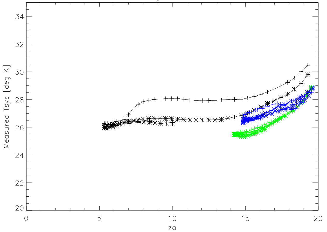
Tsys vs Za
