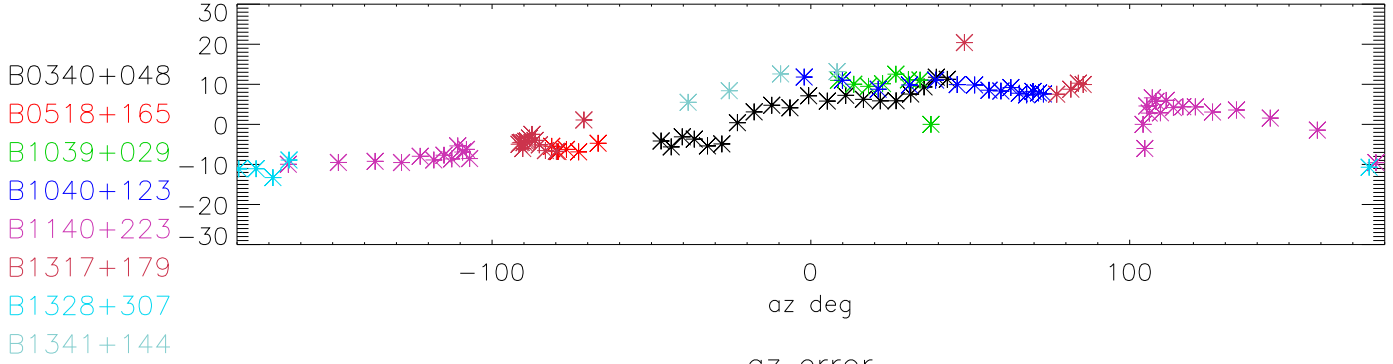
az error
