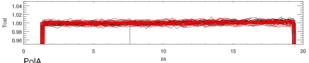
09jun11 a2130 alfaCalDeflection vs za beam0
