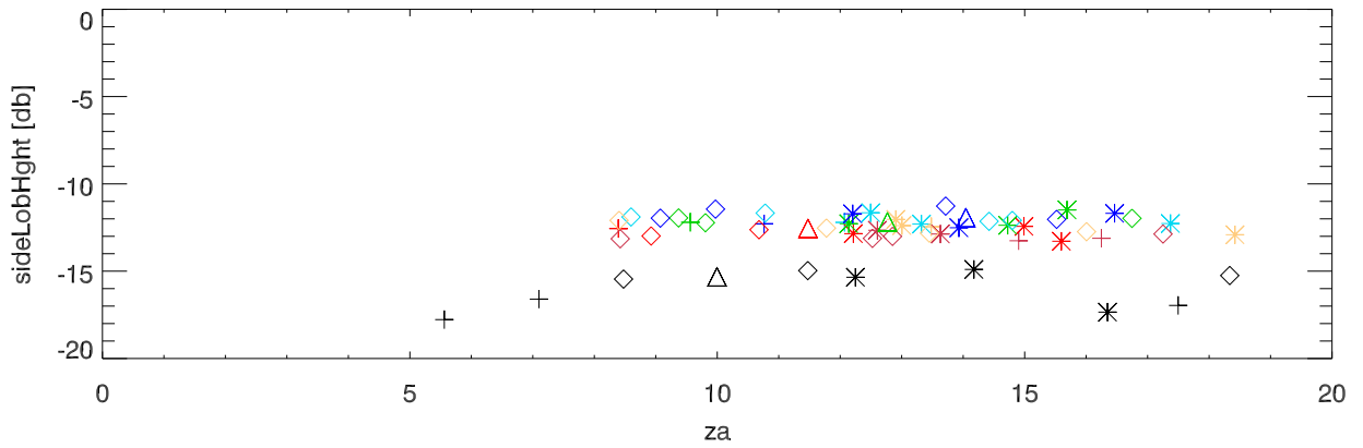
SideLobe Height
