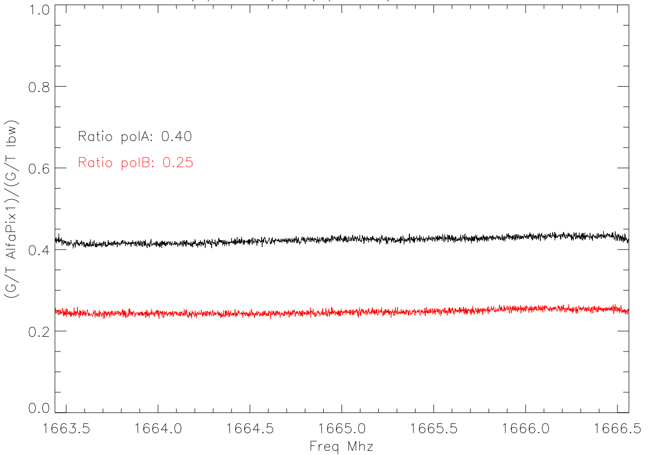
(G/T alfa) / (G/T lbw) Alfa Pixel1
