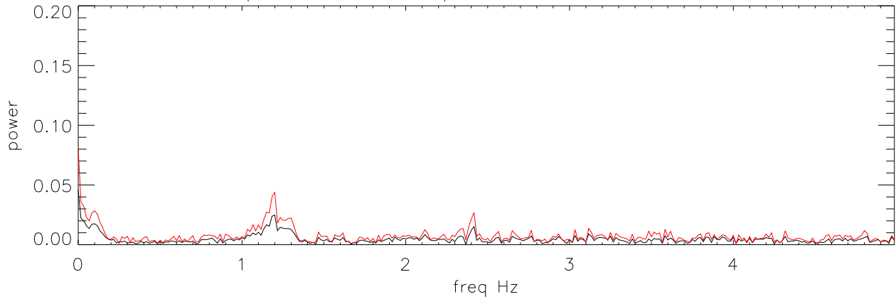
Spectrum of total power in band:1615–1785
