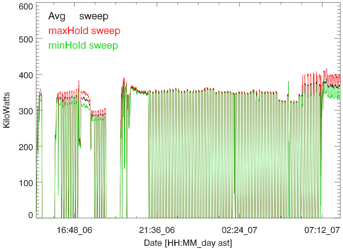
TxPwrTot. 06nov16:T2873. Juha Vierinen 5 MHz
