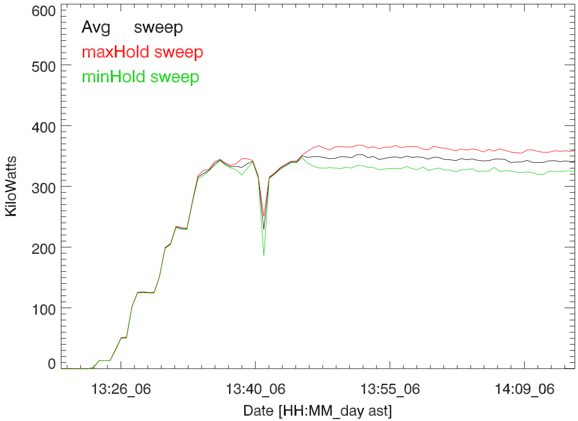
TxPwrTot. 06oct16:T2566. Paul BernHardt 8 MHz
