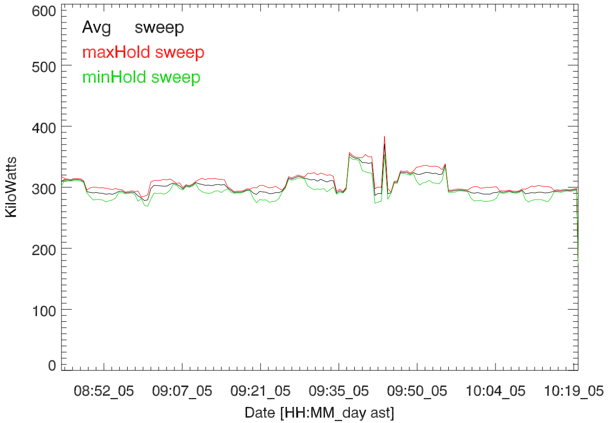
TxPwrTot. 05oct16:T2915. Salih Bostan 5 MHz
