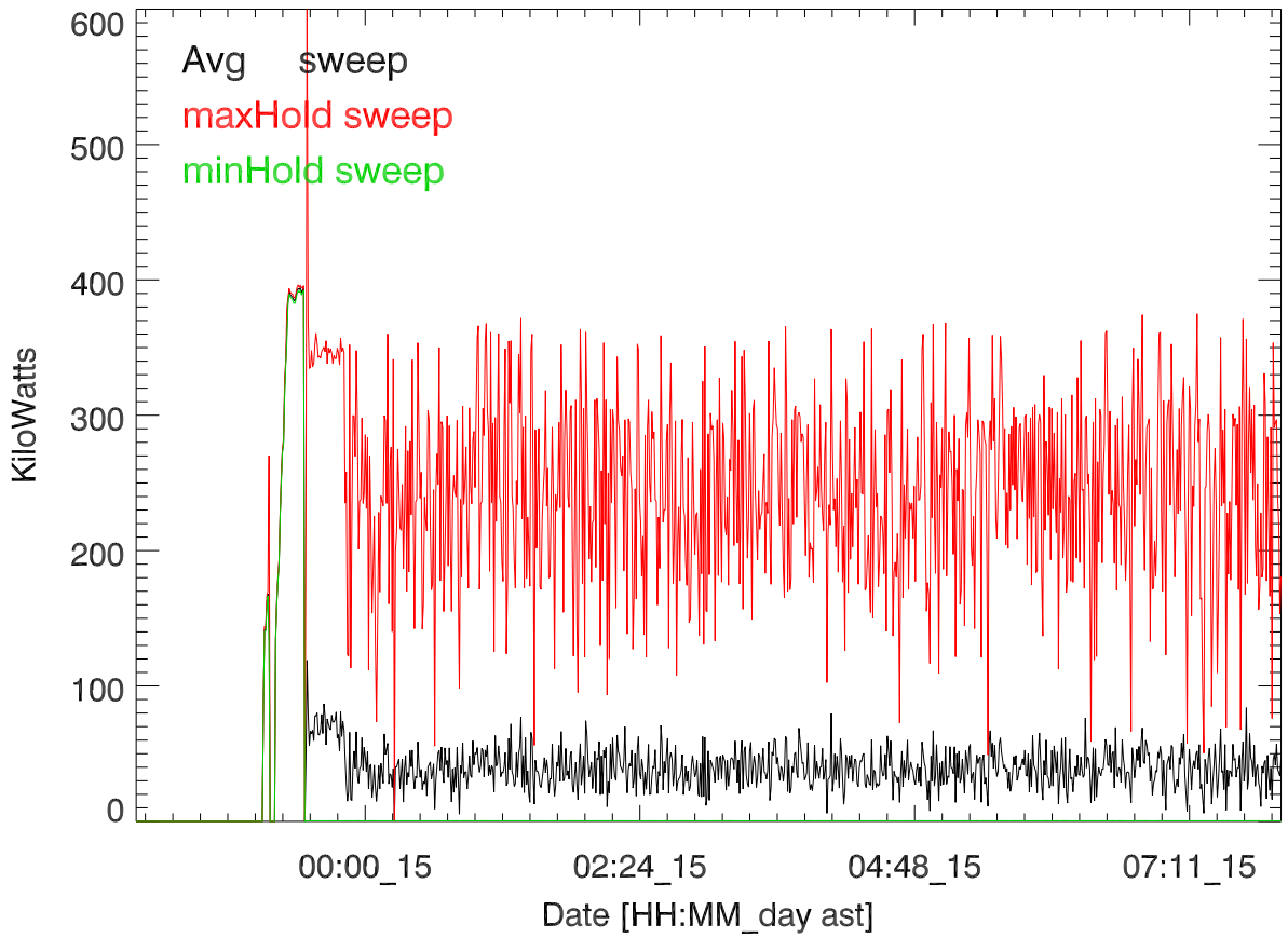
TxPwrTot. 14mar17:T2915. Salih Boston. 5 MHz
