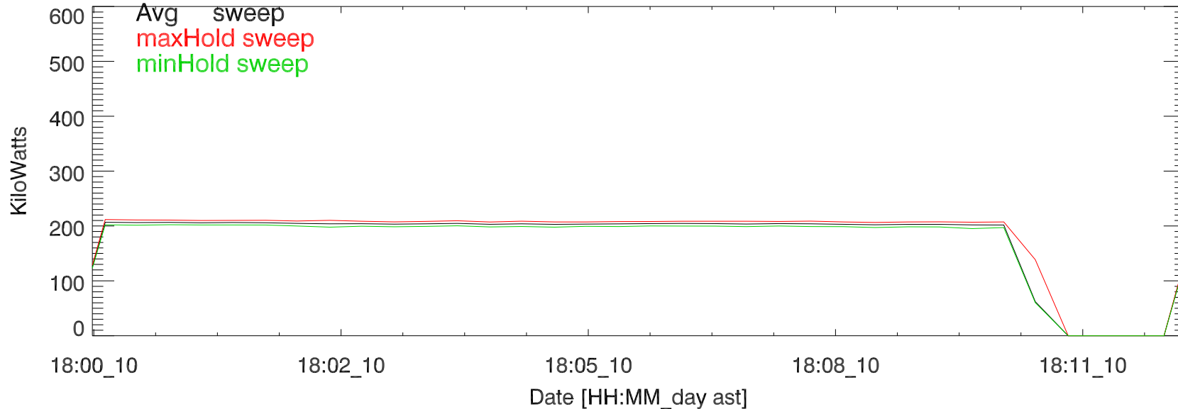
TxPwrTot. 10jun19:H3195 vladimir exp10.10 5 MHz
