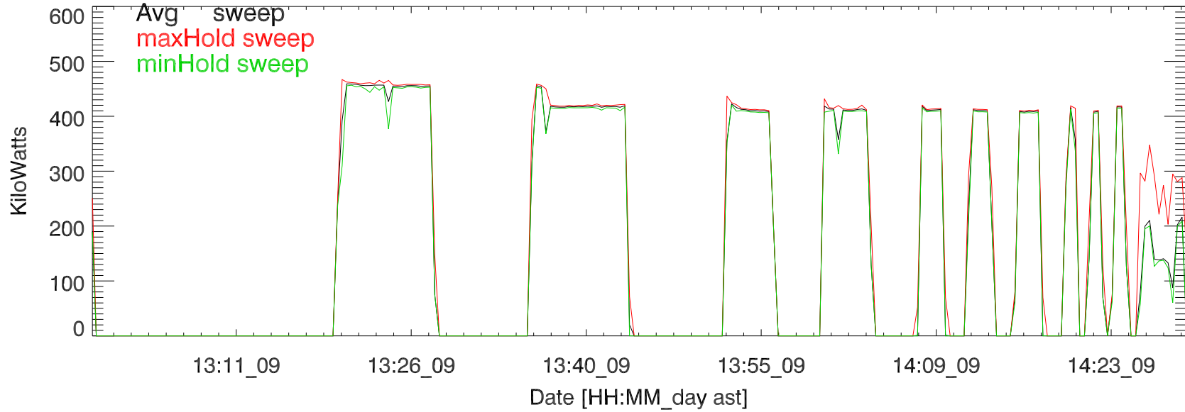
TxPwrTot. 09nov18:H3211 5 MHz
