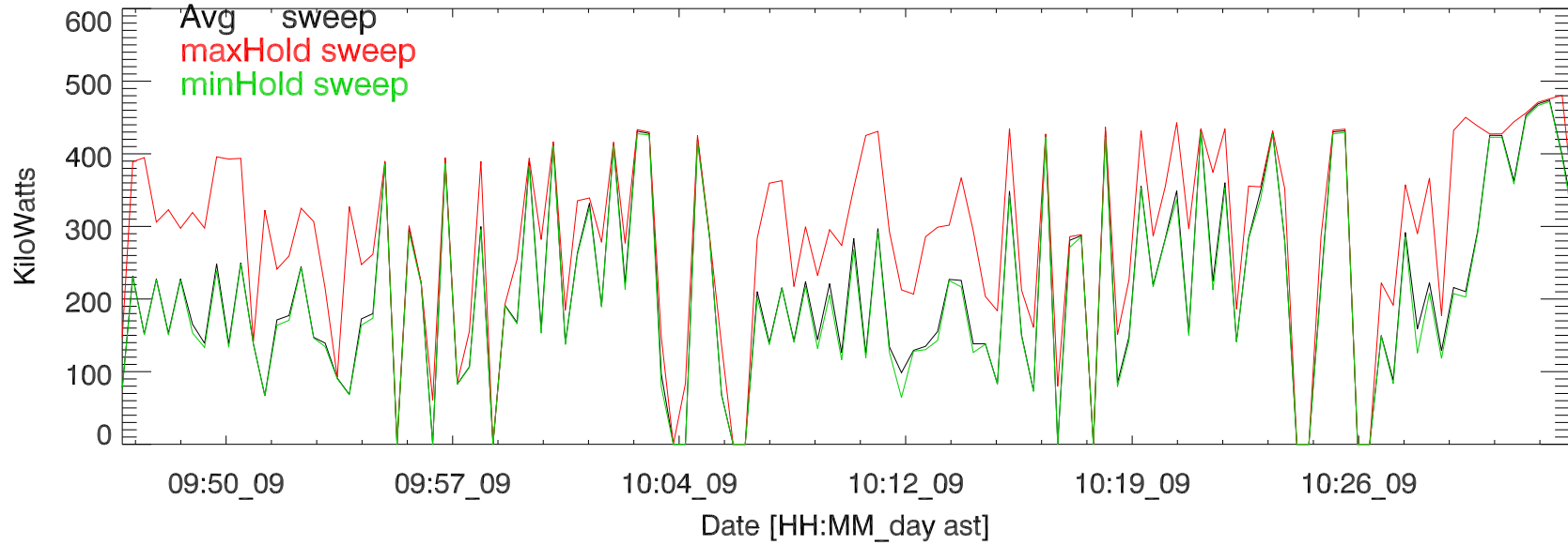
TxPwrTot. 09nov18:H3286 5 MHz
