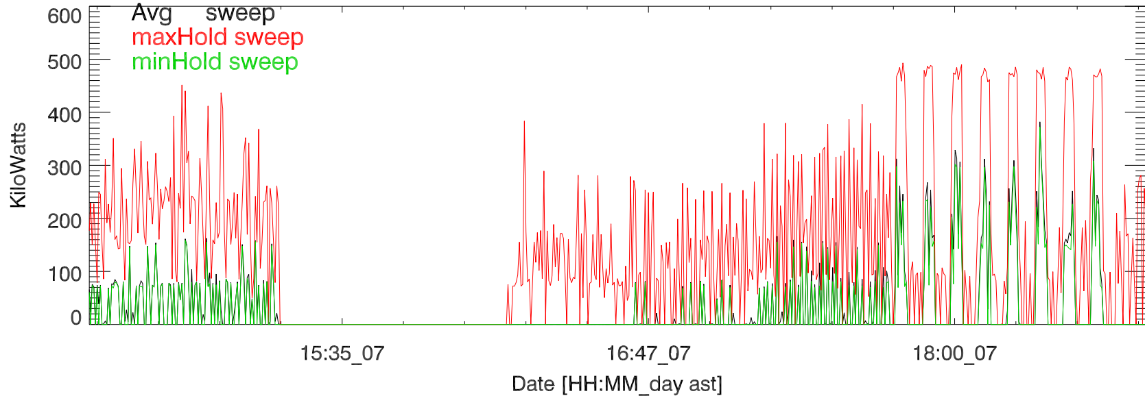
TxPwrTot. 07nov18:H3253 5 MHz
