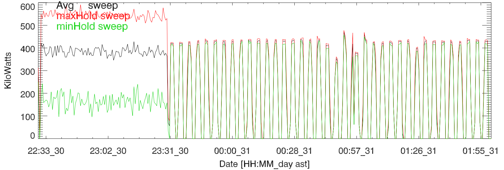
TxPwrTot. 30jul17: Jackson 5 MHz
