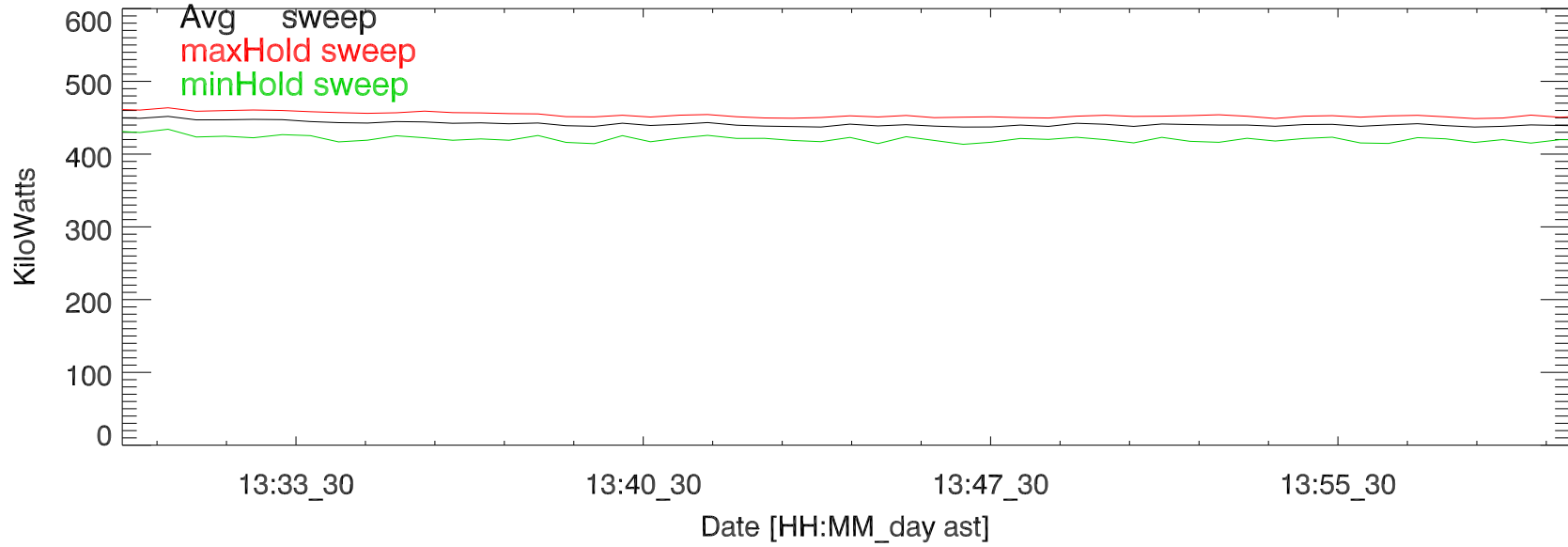
TxPwrTot. 30jul17: Paul 5 MHz
