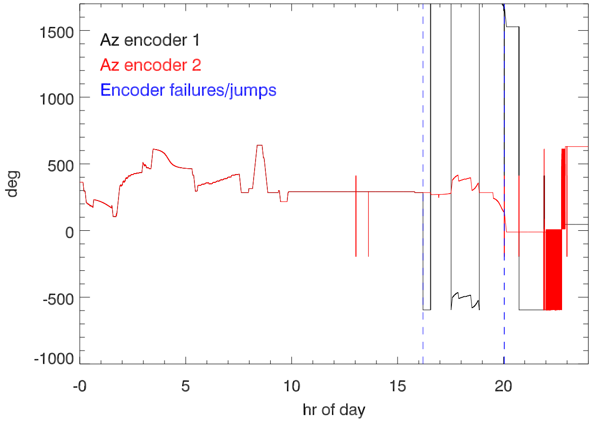
10apr17 az encoders vs hour of day
