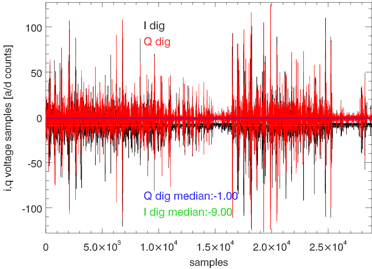
30jan18-01feb18 cad i echo i,q voltage samples
