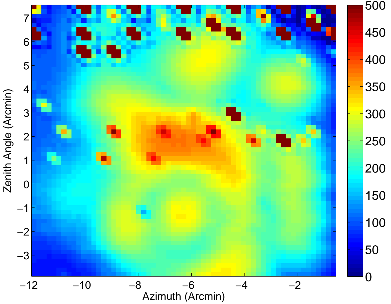
A2 Ae/Tsys Map (A2)
