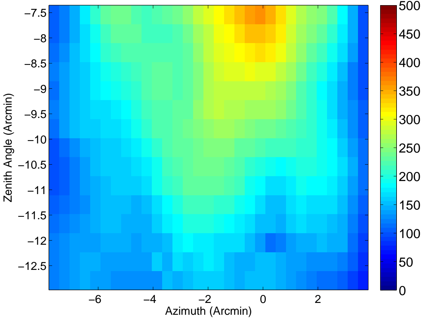
A3 Ae/Tsys Map ( z = 7.453 cm)
