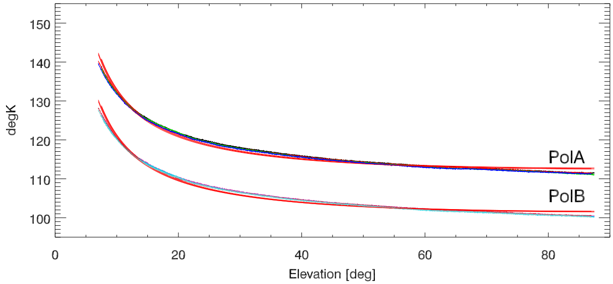
Tsys vs el and fits (Tatm=290) 8646 MHzBand
