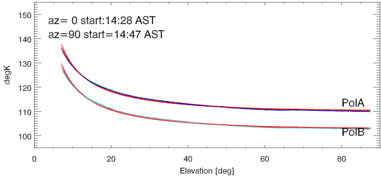
Tsys vs el and fits (Tatm=290) 8218 MHzBand
