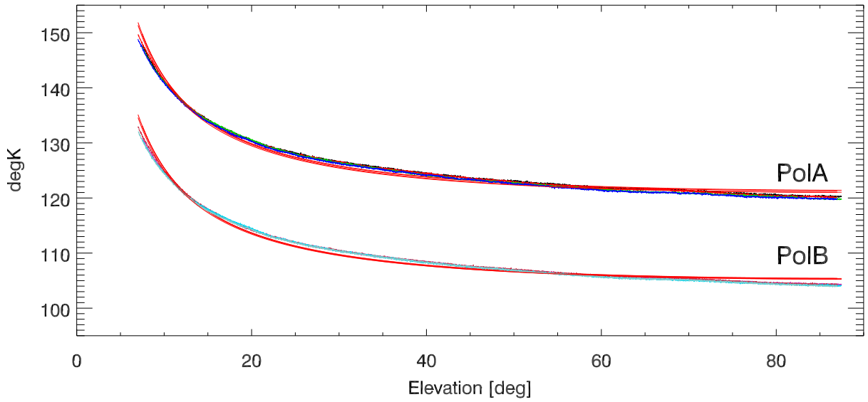
Tsys vs el and fits (Tatm=290) 9072 MHzBand
