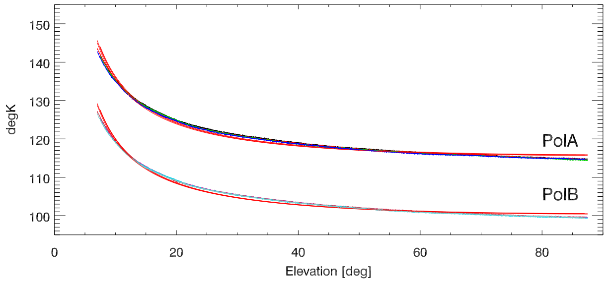
Tsys vs el and fits (Tatm=290) 8788 MHzBand
