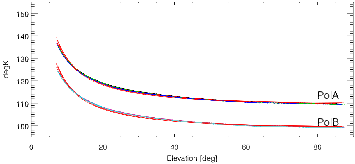
Tsys vs el and fits (Tatm=290) 8504 MHzBand
