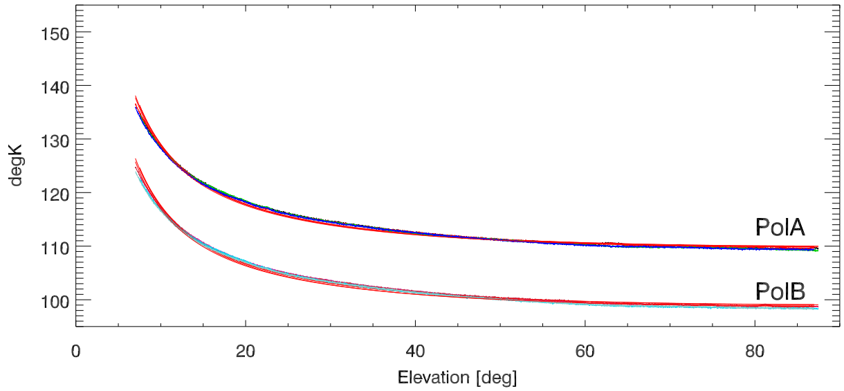
Tsys vs el and fits (Tatm=290) 8362 MHzBand
