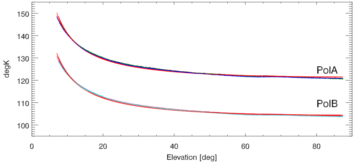
Tsys vs el and fits (Tatm=290) 8930 MHzBand
