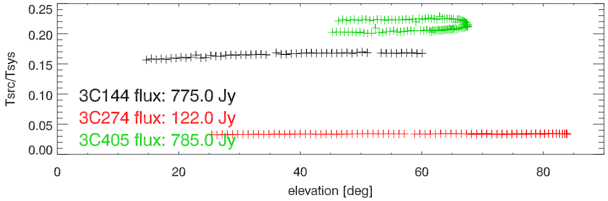
04-06apr22 sband crosses. Tsrc/Tsys vs el CFR:2270.0MHz
