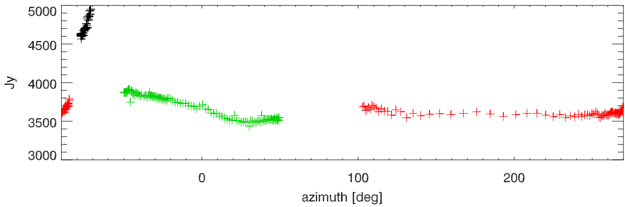
SEFD vs az
