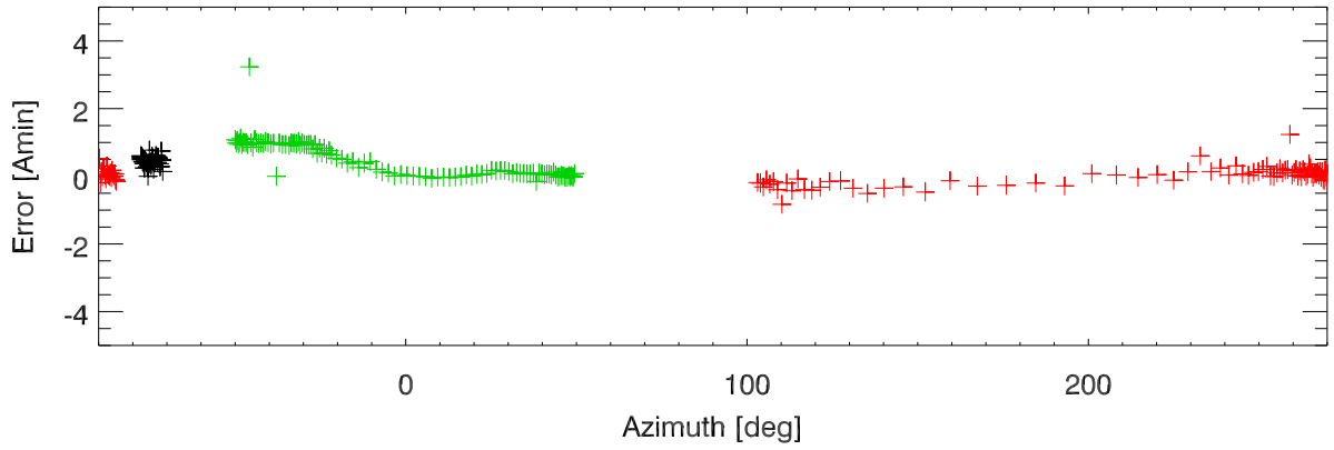
El Pointing error vs az
