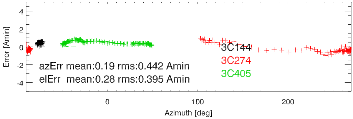
04-06apr22 Az Pointing error vs az
