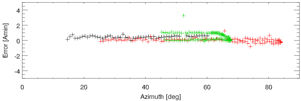
El Pointing error vs el
