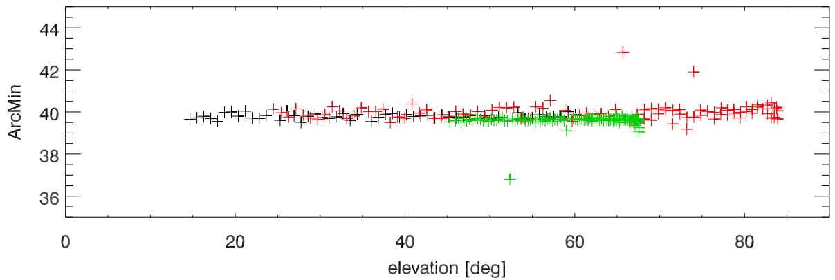
BeamWidth vs el
