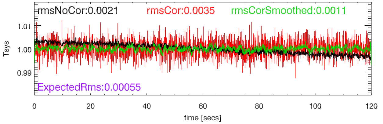
17jan22 rms 16millisec totPwr (165Mhz bw). 8218PoIA
