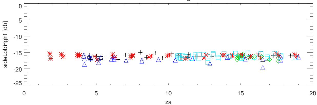
SideLobe Height
