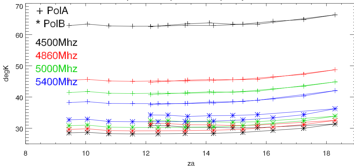
26sep12 cband polA new amp. Tsys Vs Za
