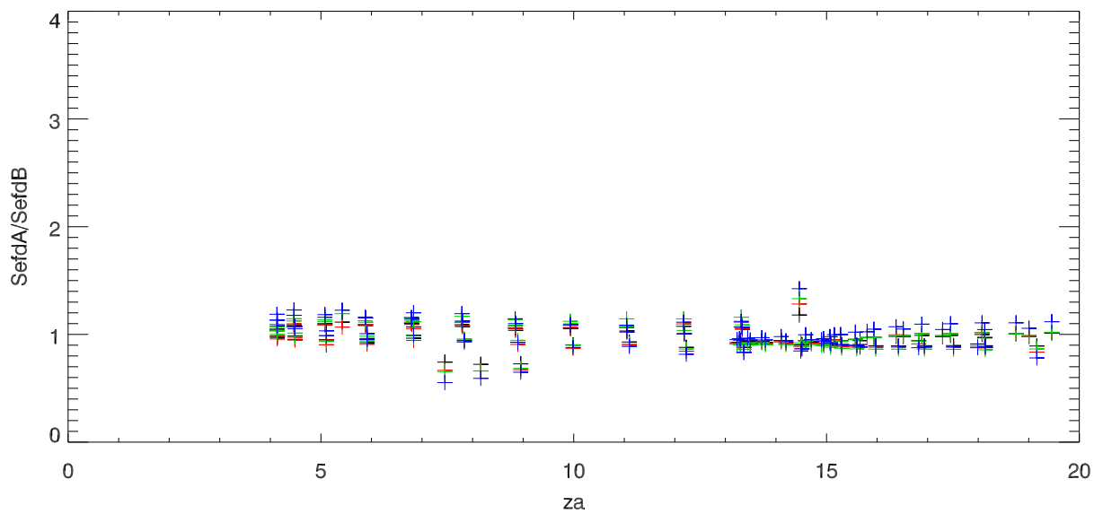
SEFD PoIA / SEFD PoIB Vs Za
