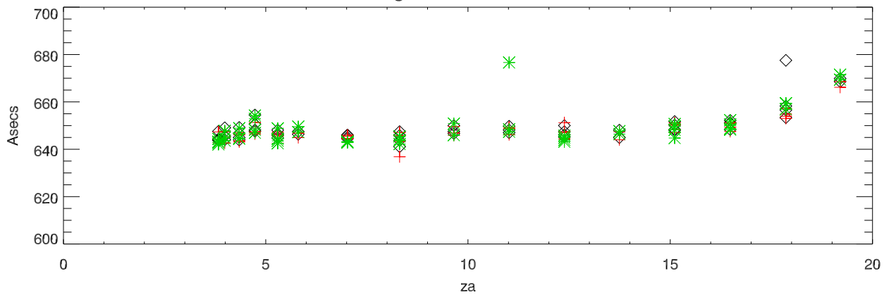
Avg Beam width vs ZA
