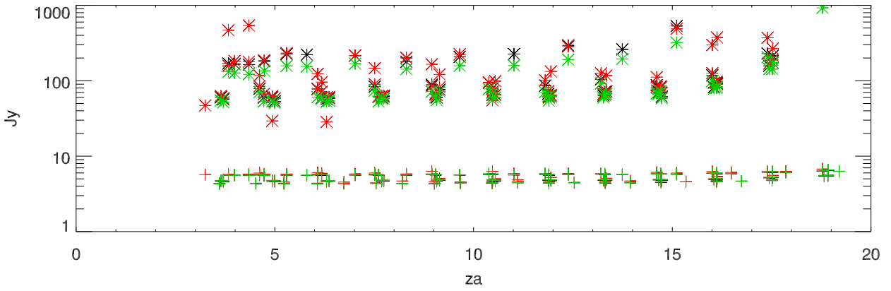
SEFD Vs Za
