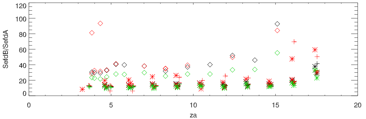
SEFD PolB /SEFD PolA Vs Za
