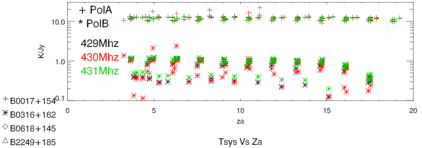
430gr jul-sep12. polA,B gain Vs Za
