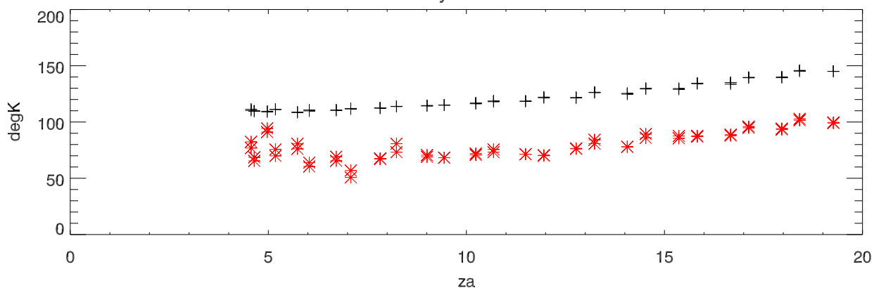
Tsys Vs Za
