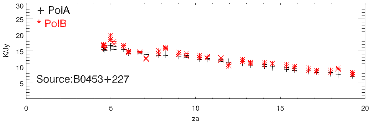
430ch 09sep15 polA,B Gain Vs Za
