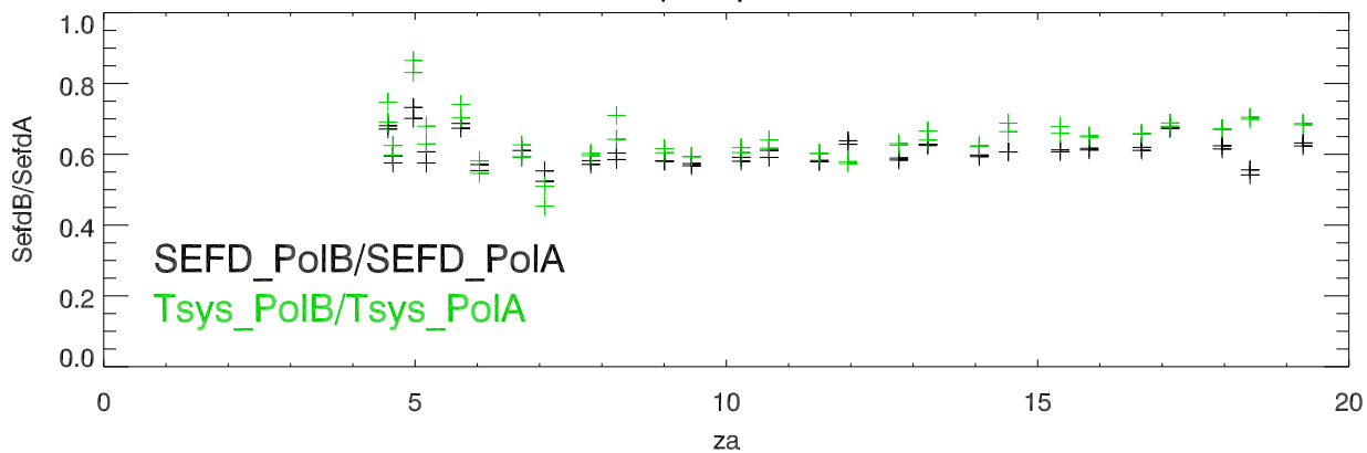
Ratios polB/polA Vs Za
