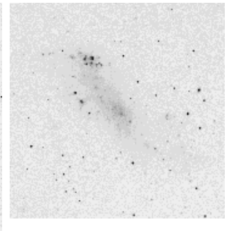
IC 2574
