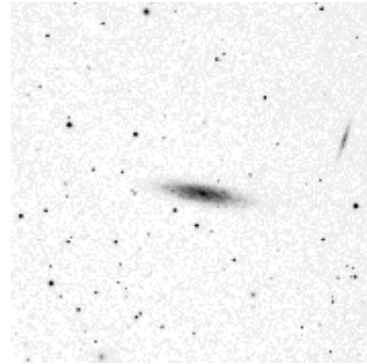
NGC 3917
