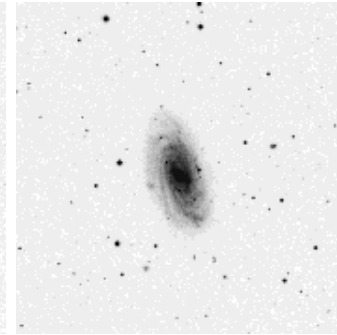
NGC 3953
