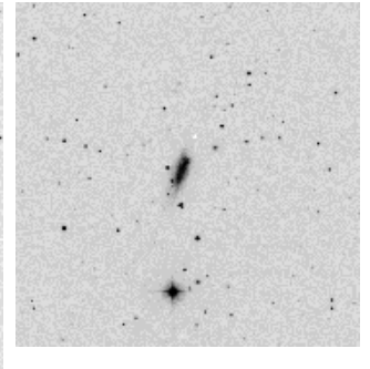
NGC 4532
