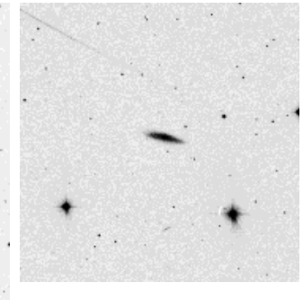
NGC 4085
