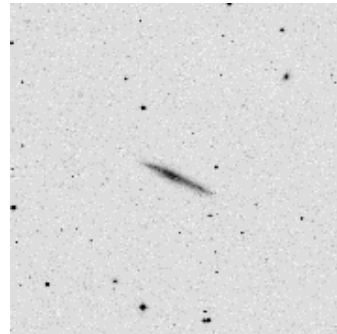
NGC 4010
