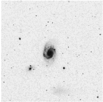
NGC 3893
