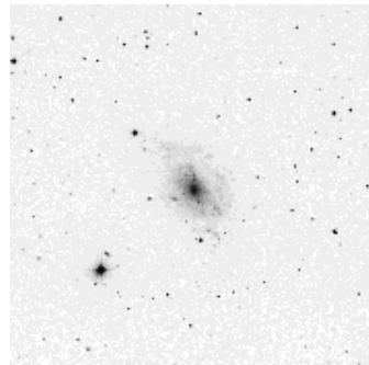
NGC 5585
