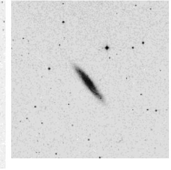
NGC 3877
