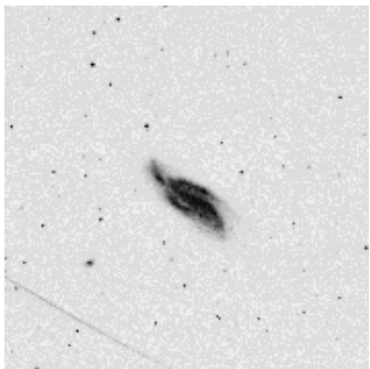
NGC 4088
