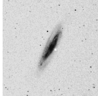
NGC 4192
