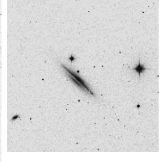
NGC 4217
