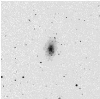
NGC 5204
