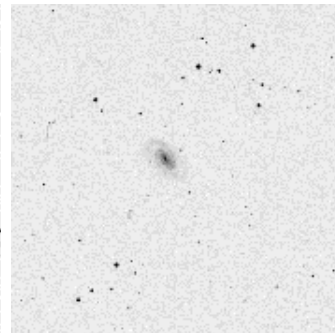
IC 769
