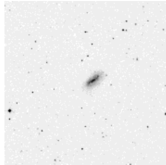
NGC 4498
