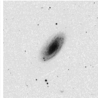
NGC 4501
