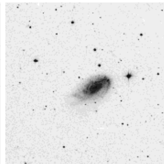
NGC 4654
