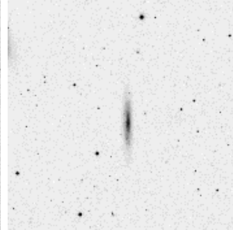
NGC 4206
