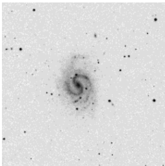
NGC 4535
