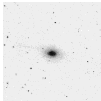
NGC 4651
