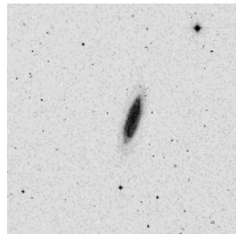
NGC 4100
