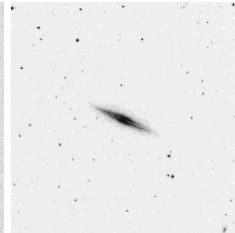
NGC 4013
