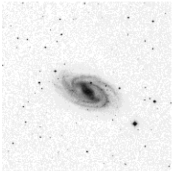
NGC 3992
