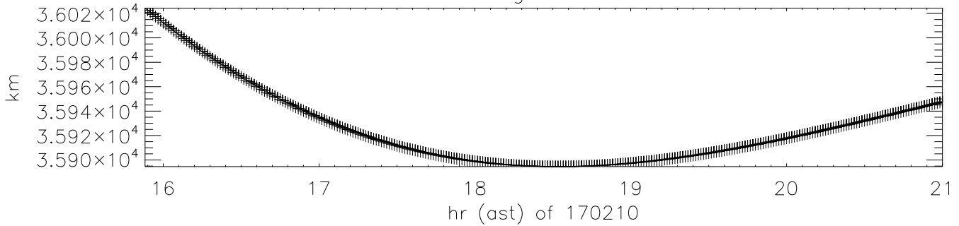
Echo return modulo 13.0ms ipp
