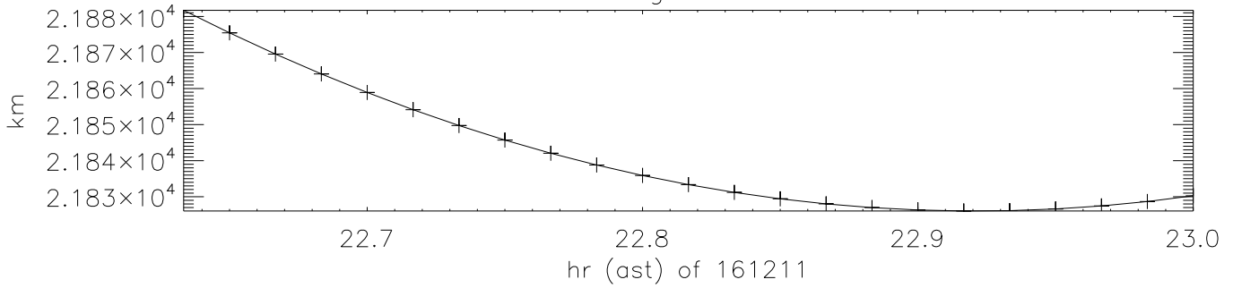
Echo return modulo 11.1ms ipp
