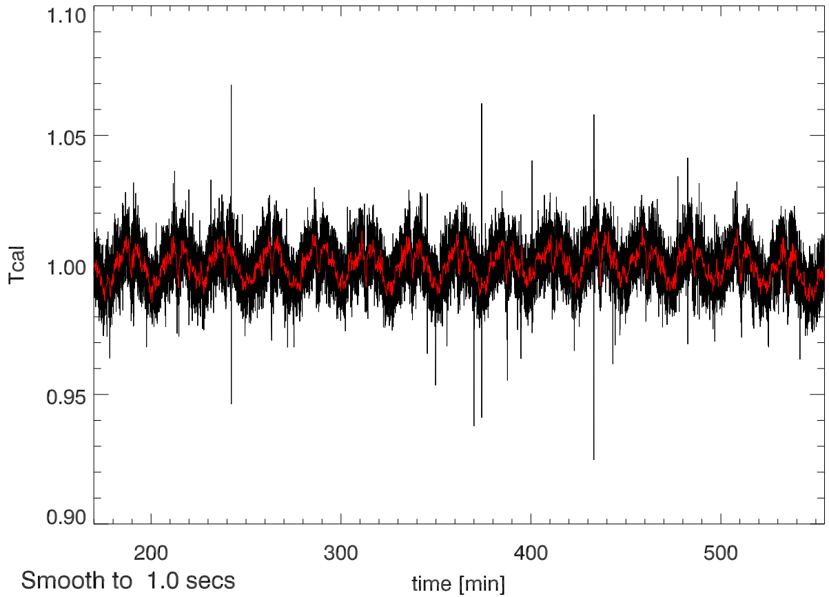
29jan13 calOn - calOff Beam3A SigA: 0.014
